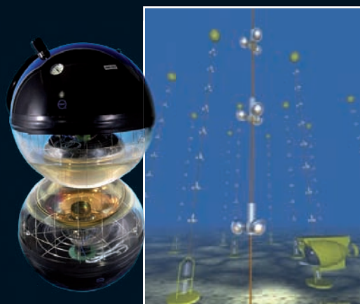
Antarès. Un dispositif immergé au fond de la Méditerranée capte la lumière émise par des particules ayant interagi avec des neutrinos de très haute énergie d'origine cosmique qui ont traversé la Terre.
